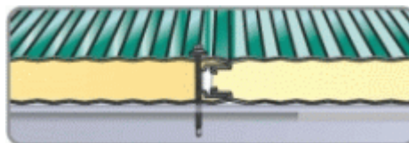
Detaliu de fixare
