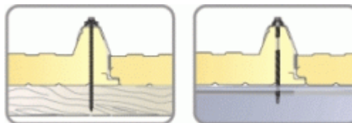
Detaliu de fixare
