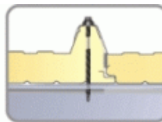
Detaliu de fixare
